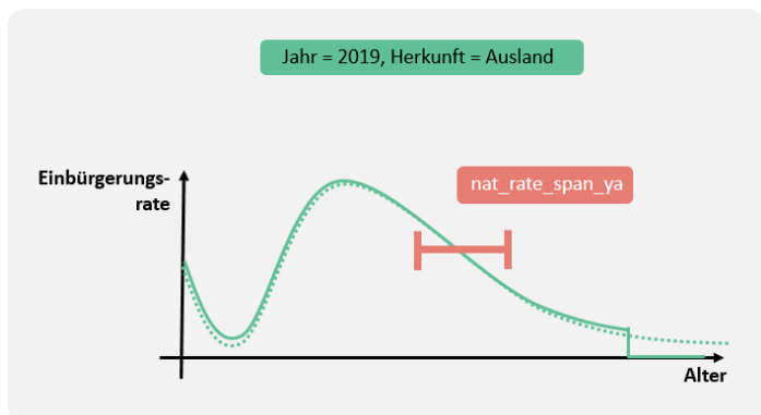
Abbildung 41: Einbürgerungsrate glätten
